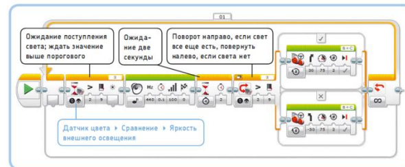
Рис. 3.17. Программа MorseCode. И первый блок Ожидание, и блок Переключатель находится в режиме Датчик цвета → Сравнение → Яркость внешнего освещения
