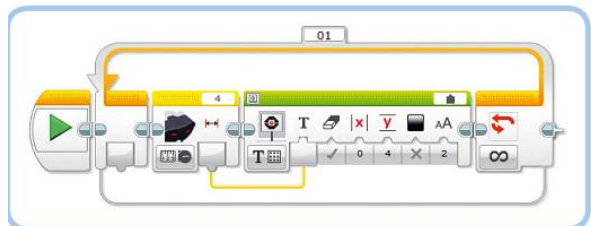
Рис. 14.17. Программа DisplayNumeric
